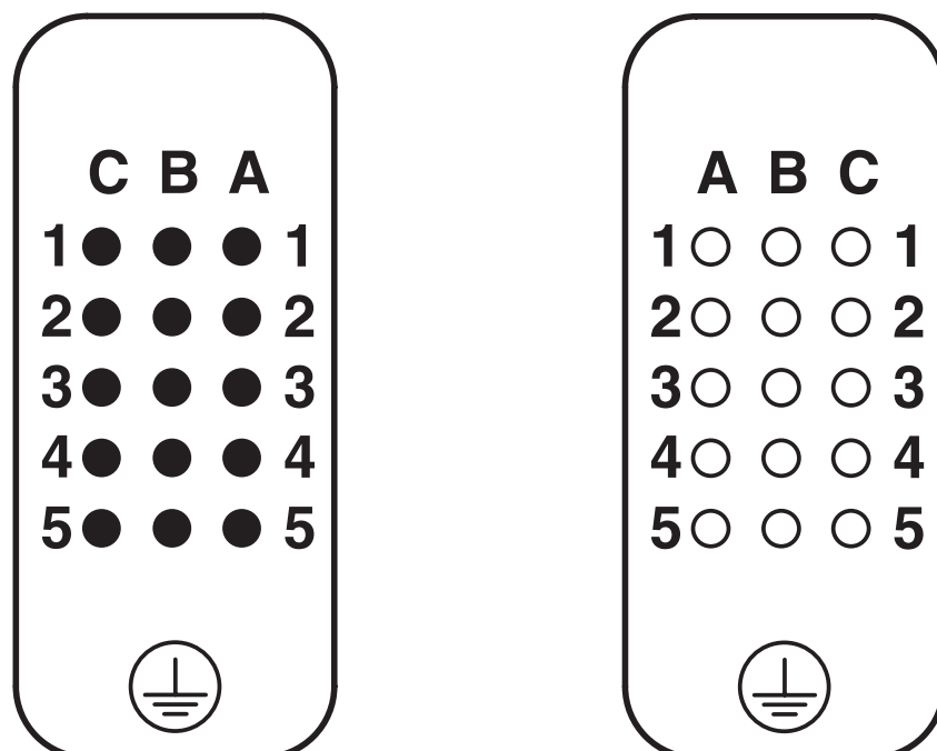
Układ styków - widok od strony przyłączy: lewy wtyk, prawe gniazdo
