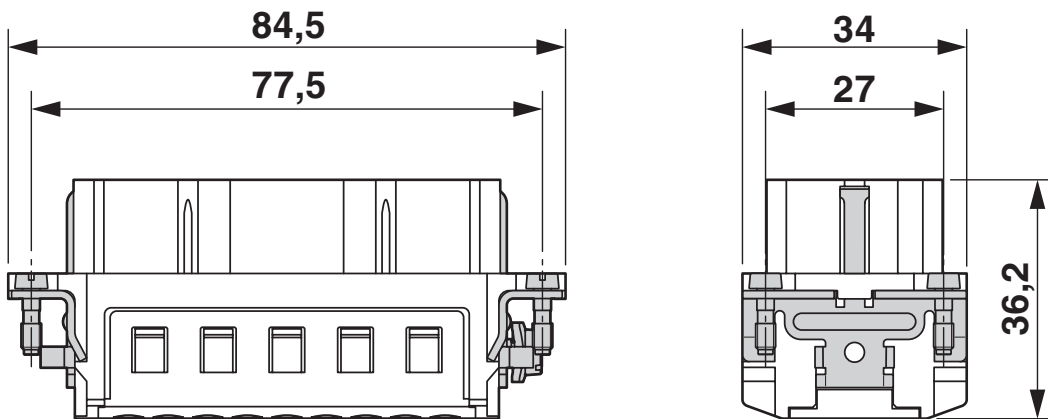
Rysunek wymiarowy
