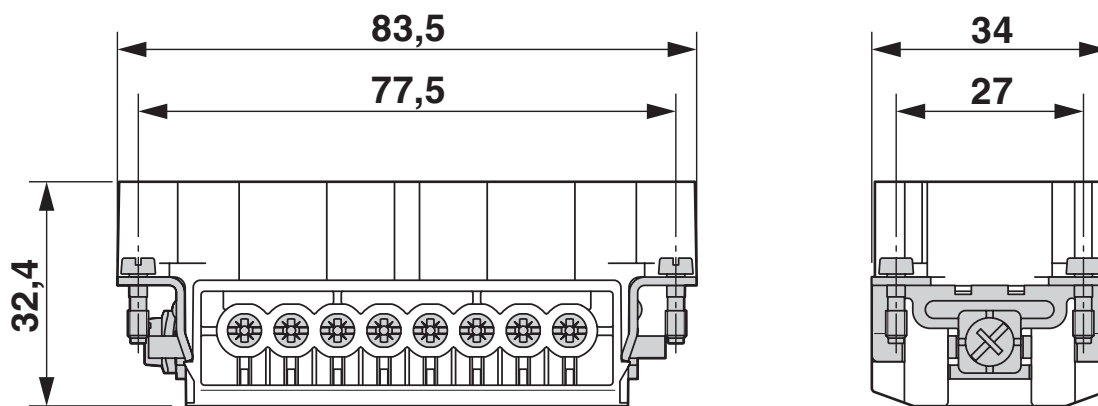
Rysunek wymiarowy
