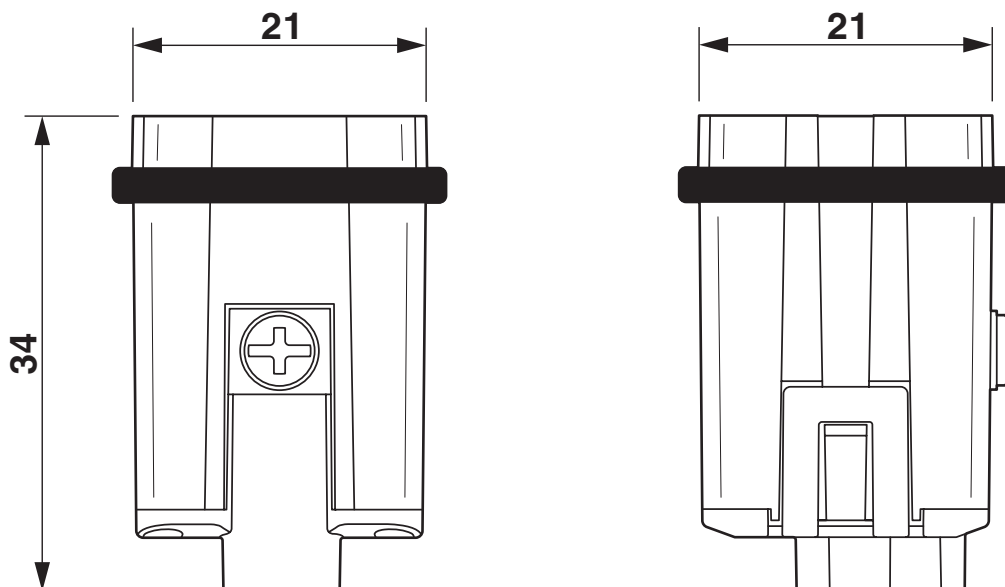
Rysunek wymiarowy
