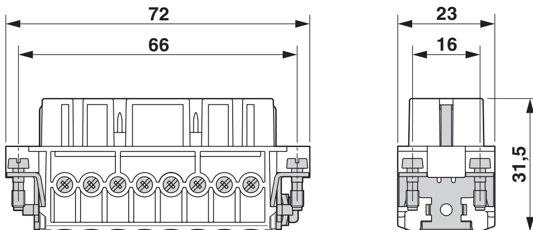
Rysunek wymiarowy
