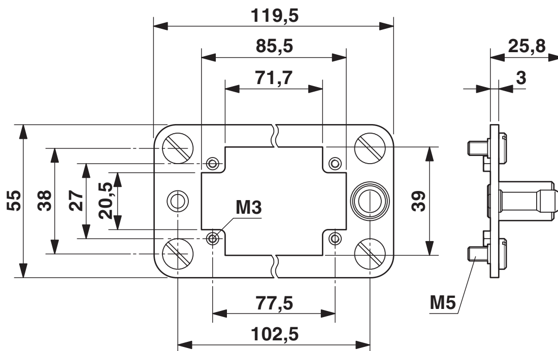
Rysunek wymiarowy
