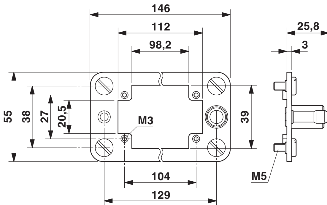
Rysunek wymiarowy
