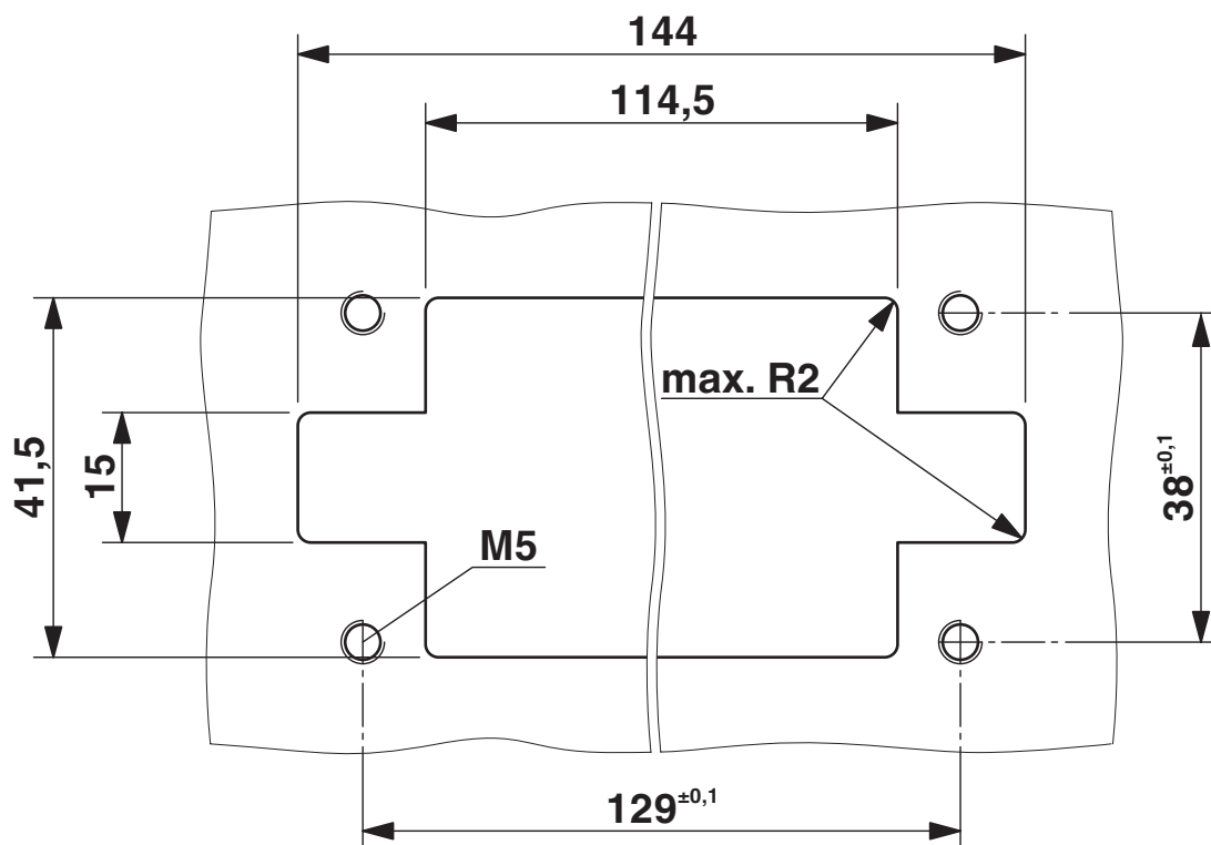
Rysunek wymiarowy
