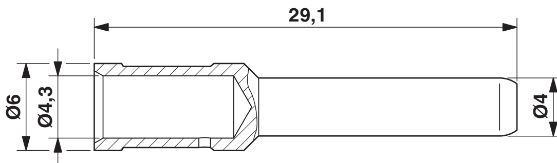
Rysunek wymiarowy
