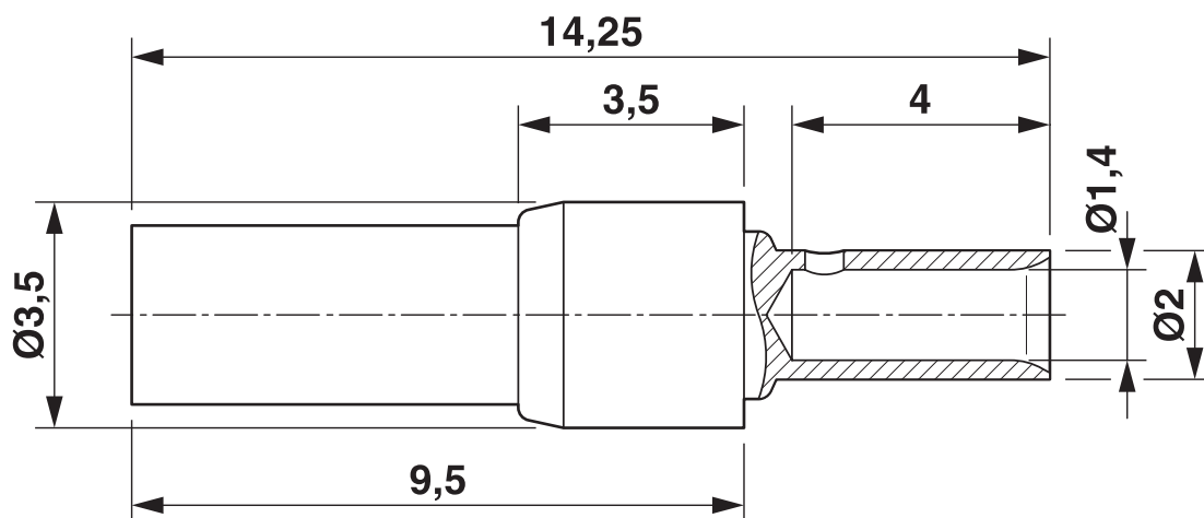
Rysunek wymiarowy
