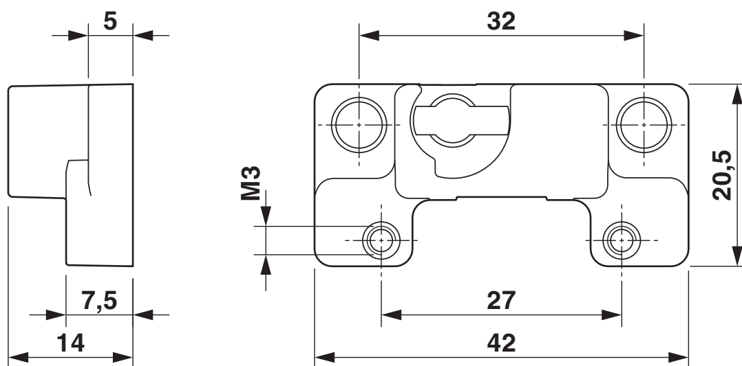
Rysunek wymiarowy
