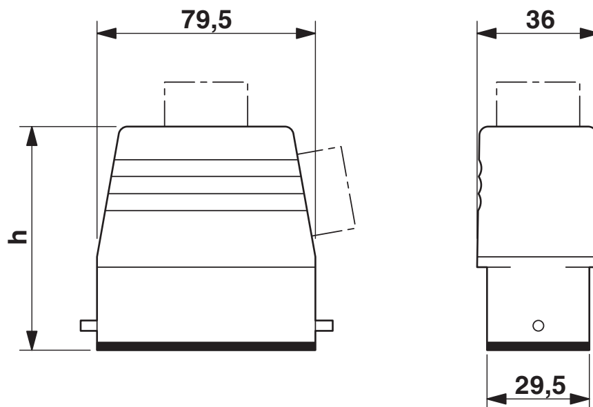
Rysunek wymiarowy
