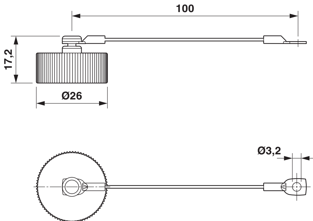
Rysunek wymiarowy
