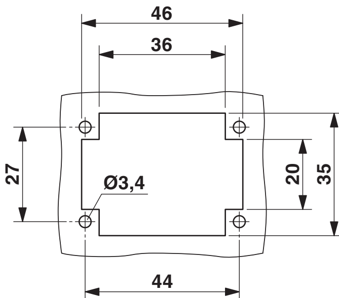
Wycięcie montażowe przy zastosowaniu bez obudowy
