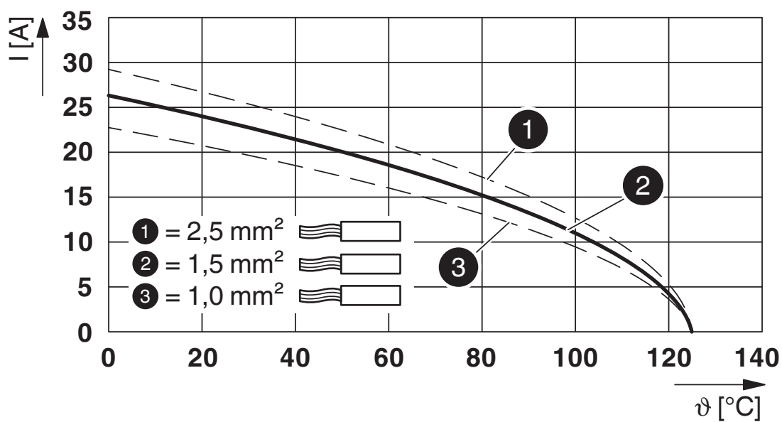
Wykres obniżenia parametrów znamionowych dla linek
