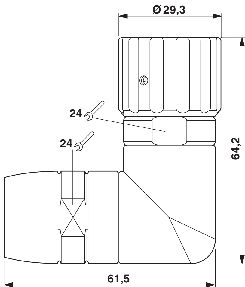
Rysunek wymiarowy
