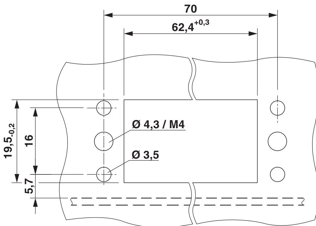
Rysunek wymiarowy
