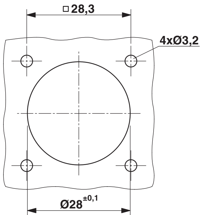
Rysunek wymiarowy
