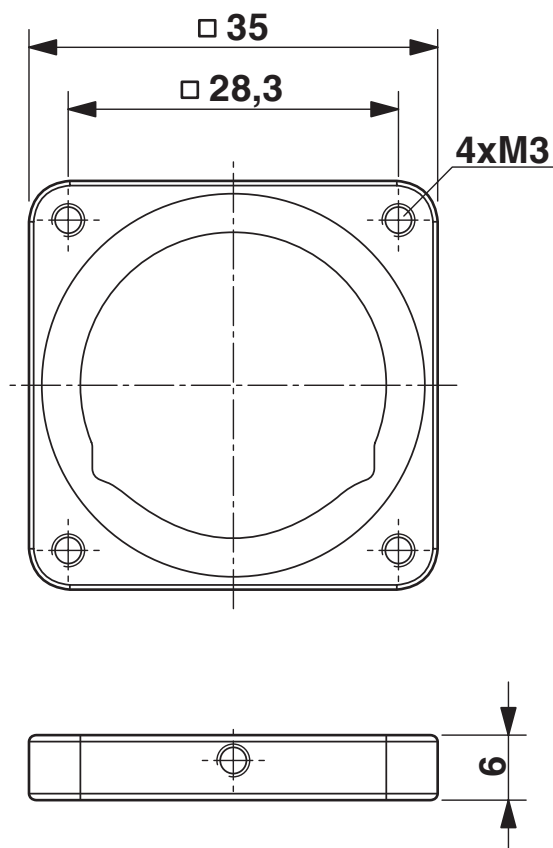
Rysunek wymiarowy
