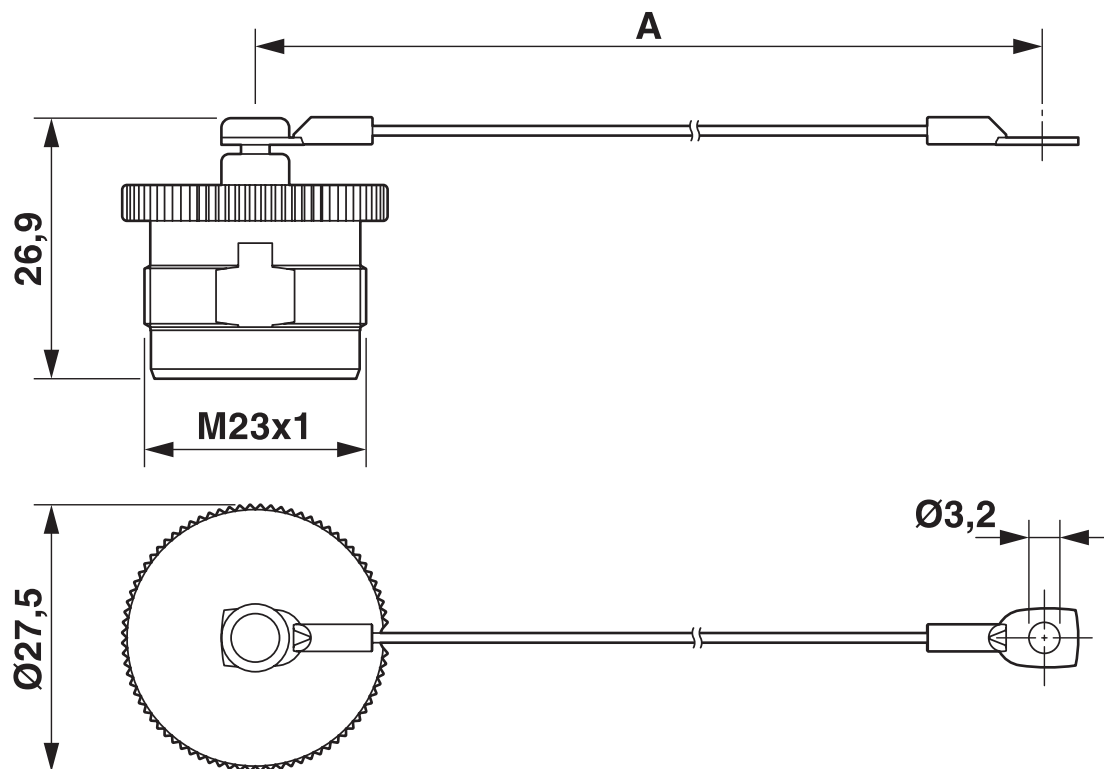
Rysunek wymiarowy
