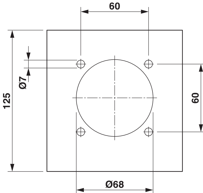
Rysunek wymiarowy
