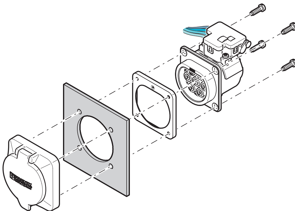
Rysunek schematyczny
