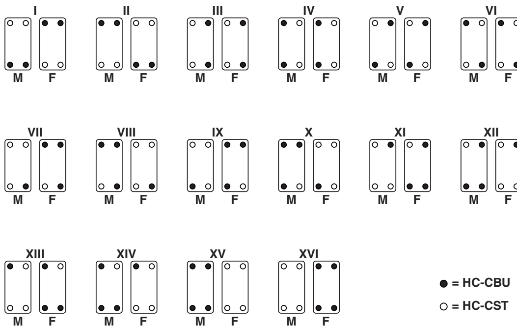
Schemat
