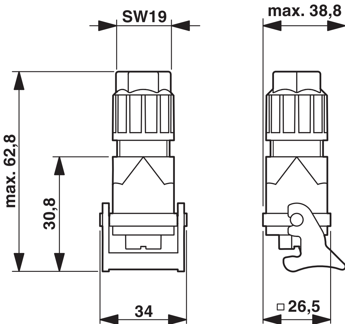
Rysunek wymiarowy
