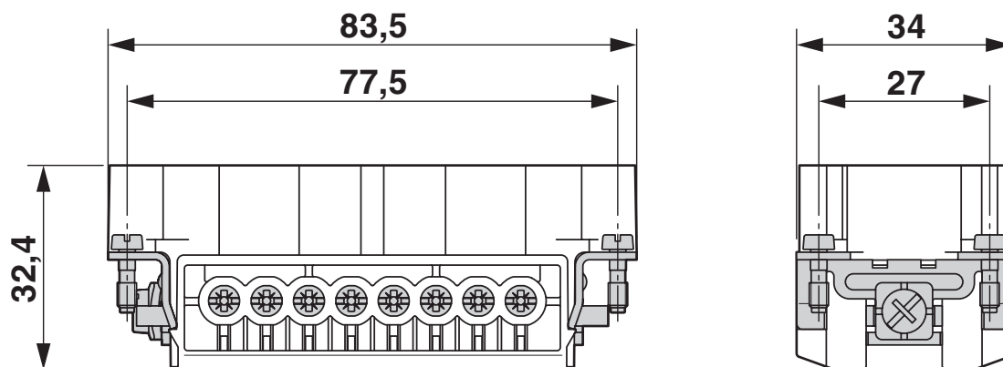
Rysunek wymiarowy
