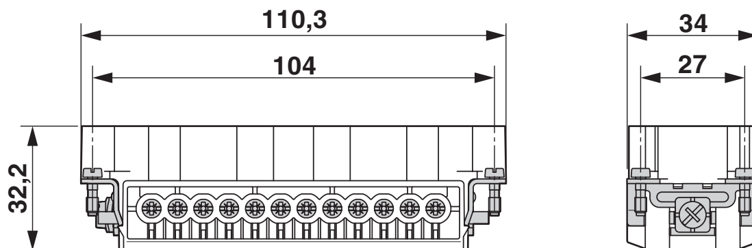
Wkładka styków męskich
