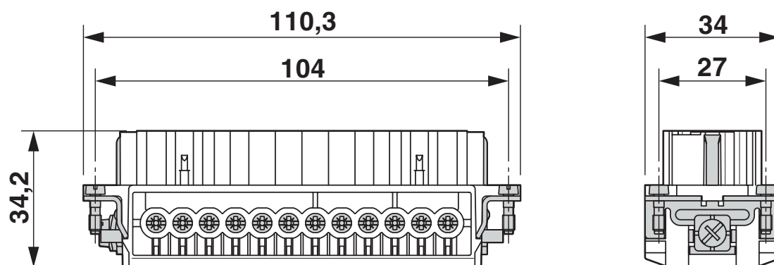
Rysunek wymiarowy
