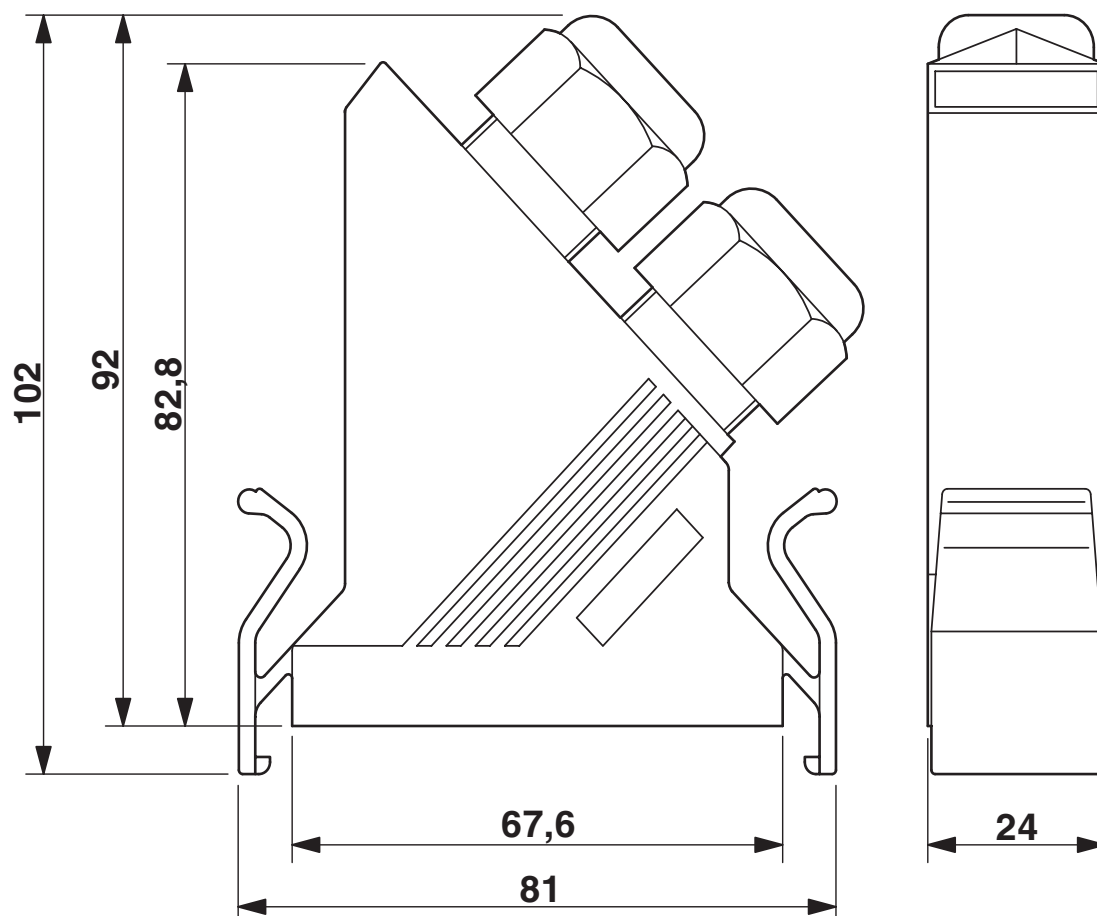
Rysunek wymiarowy
