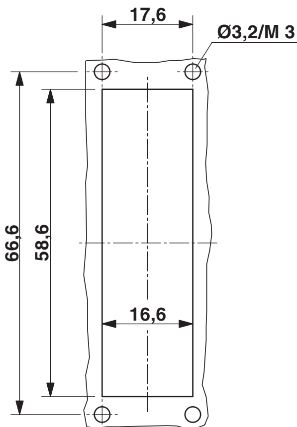
Rysunek wymiarowy
