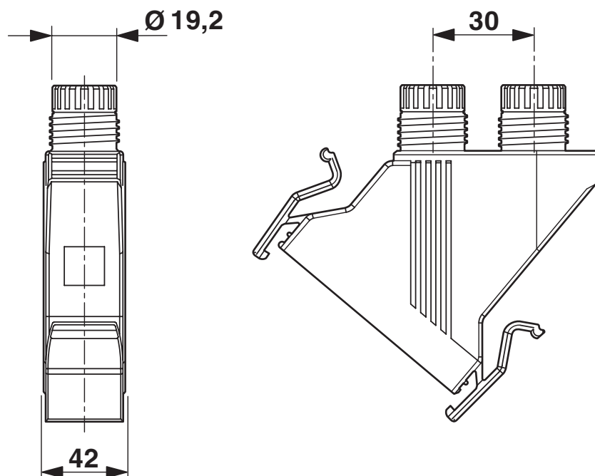
Rysunek wymiarowy
