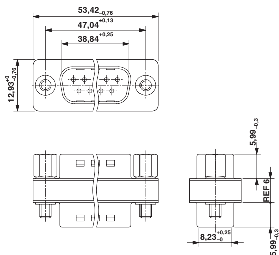
Rysunek wymiarowy
