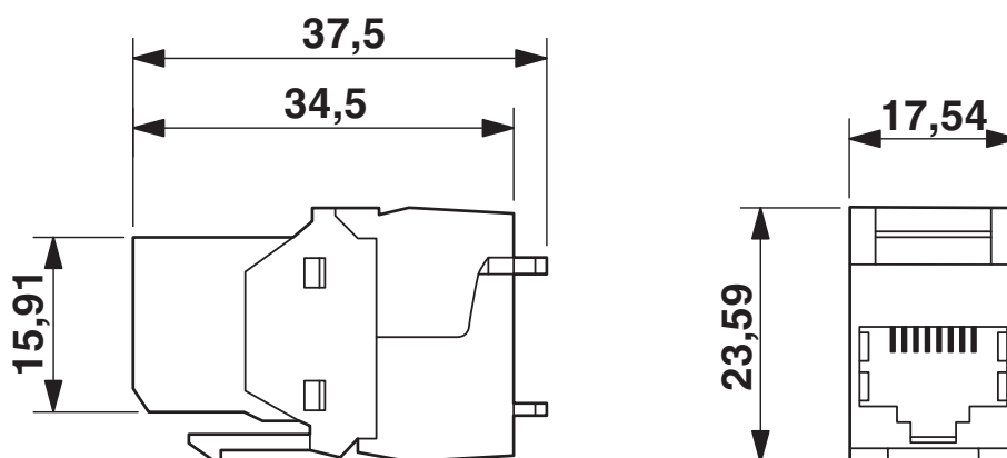
Rysunek wymiarowy
