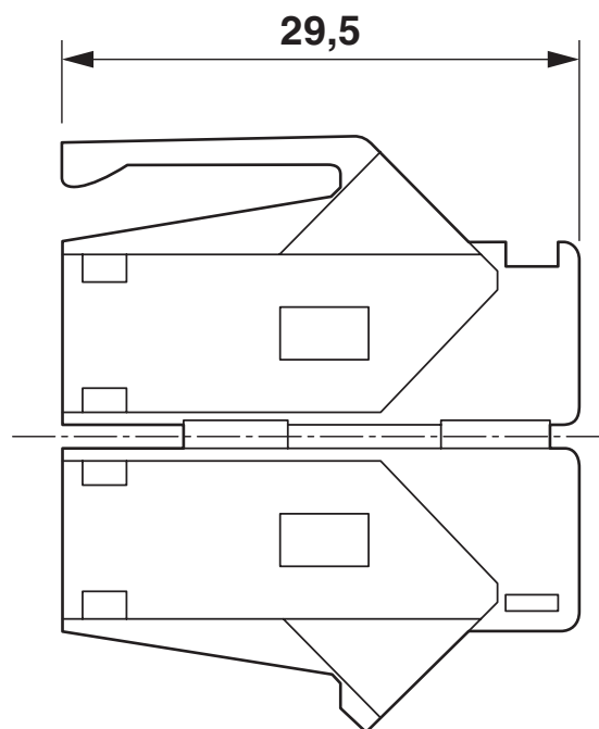
Rysunek wymiarowy
