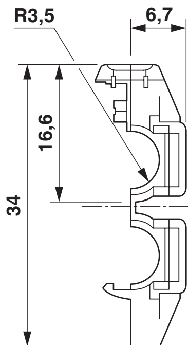
Tuleja usztywniająca RJ45
