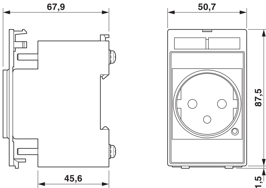
Rysunek wymiarowy
