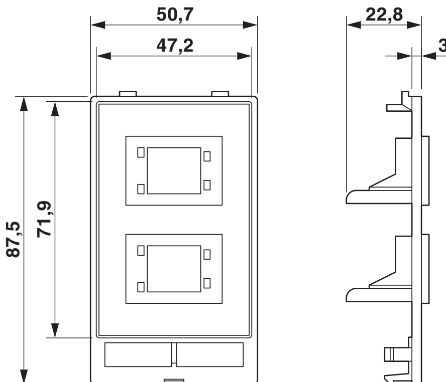
Rysunek wymiarowy
