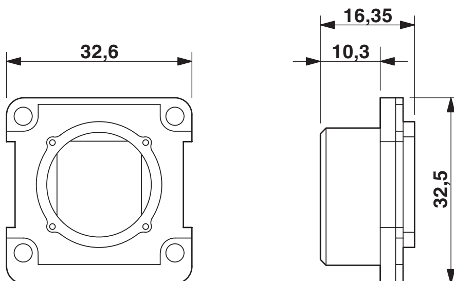
Rysunek wymiarowy
