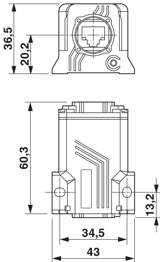
Rysunek wymiarowy
