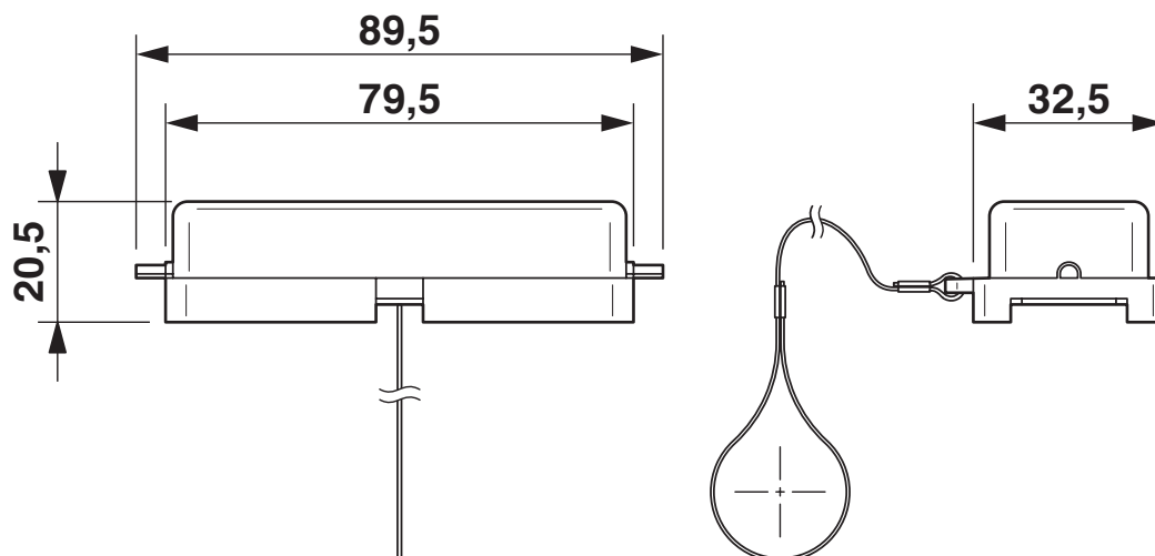
Rysunek wymiarowy
