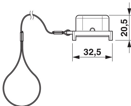
Rysunek wymiarowy
