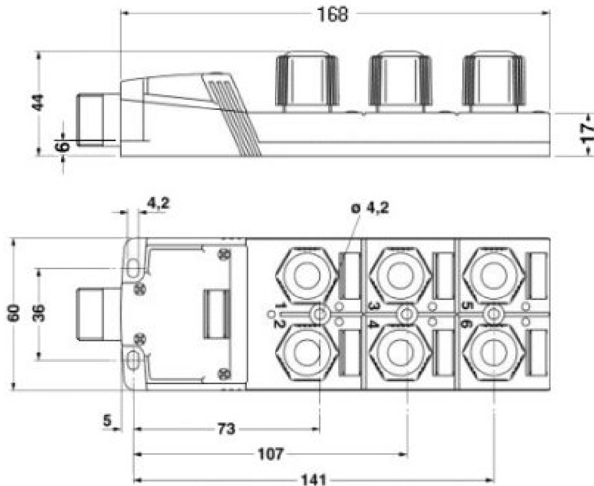
Rysunek wymiarowy
