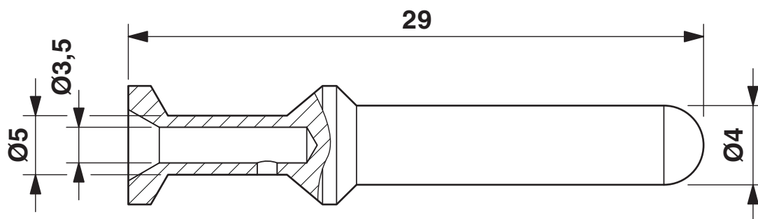
Rysunek wymiarowy
