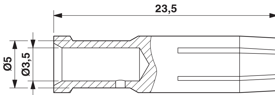
Rysunek wymiarowy
