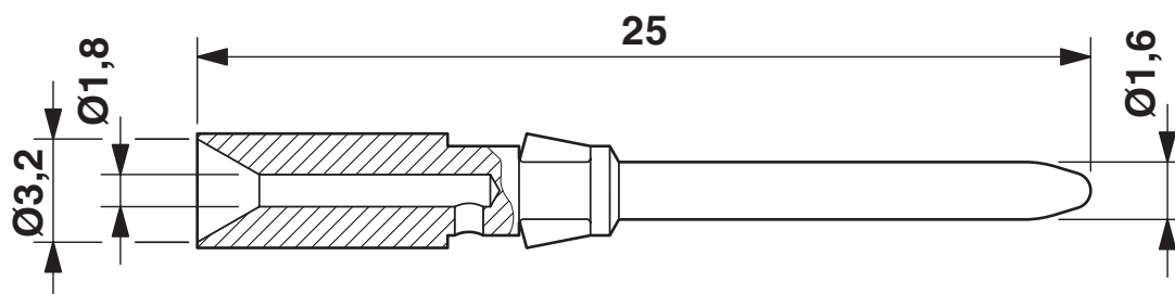
Rysunek wymiarowy
