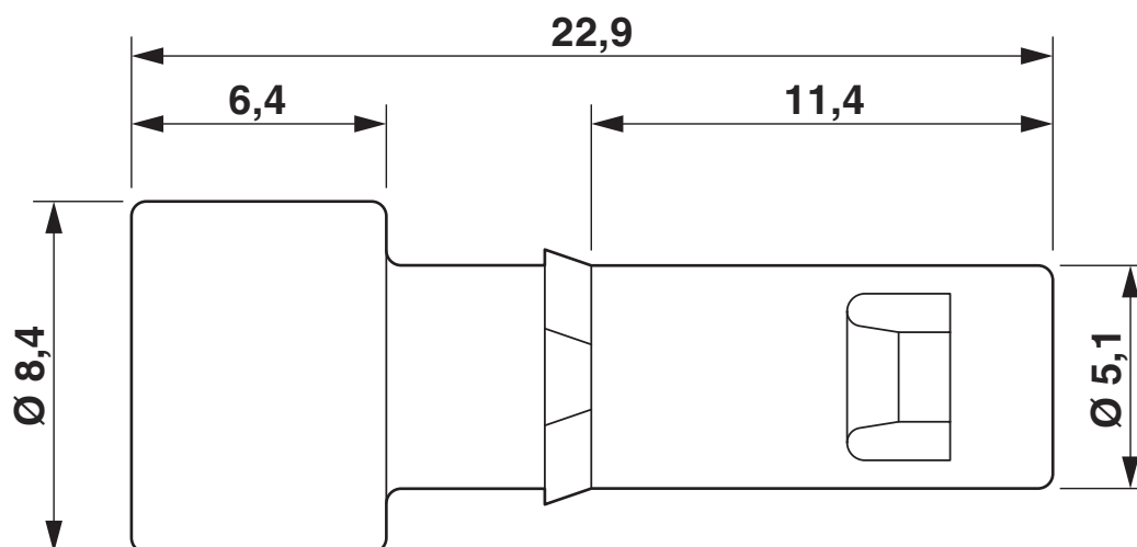
Rysunek wymiarowy
