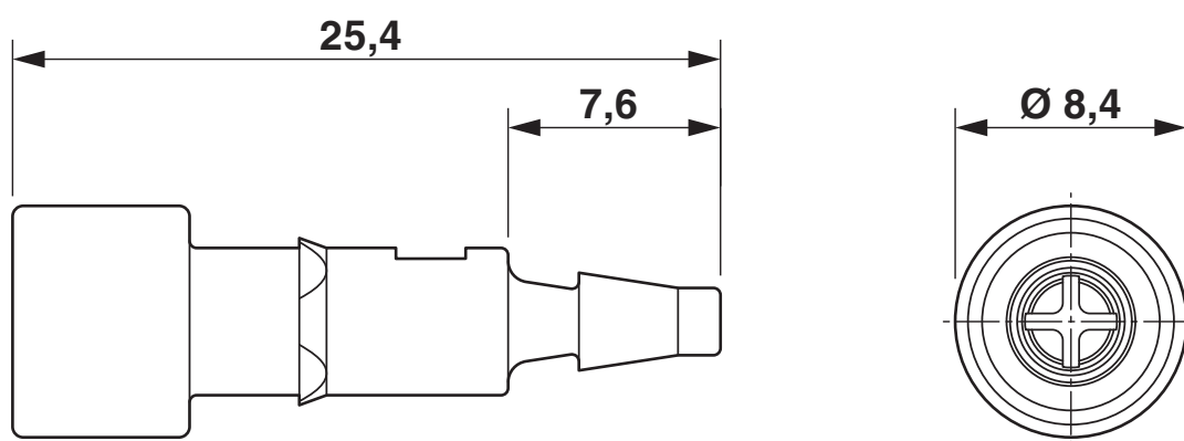
Rysunek wymiarowy
