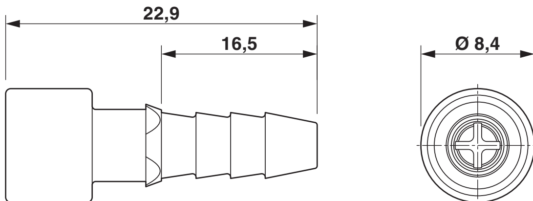
Rysunek wymiarowy
