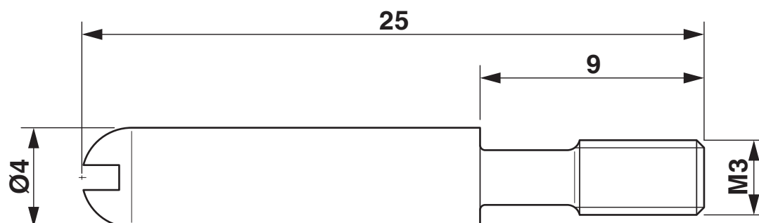
Rysunek wymiarowy
