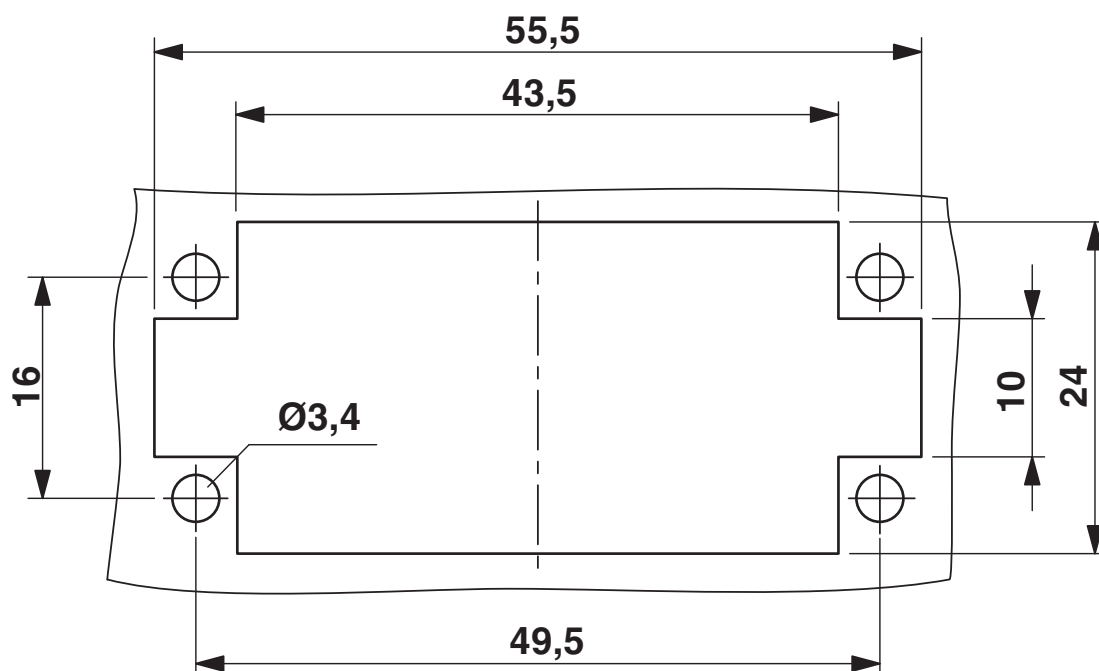
Wycięcie montażowe przy zastosowaniu bez obudowy
