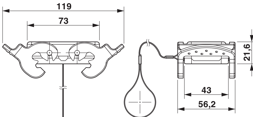
Rysunek wymiarowy
