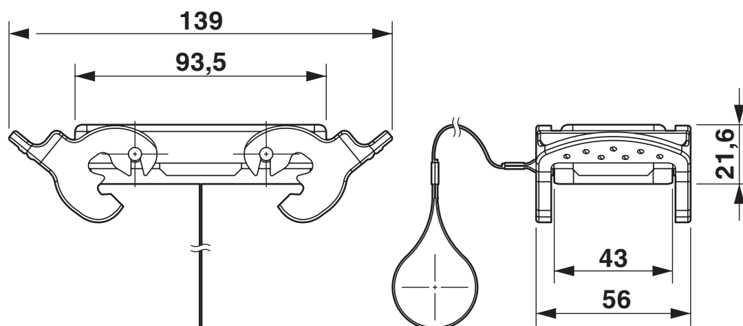
Rysunek wymiarowy
