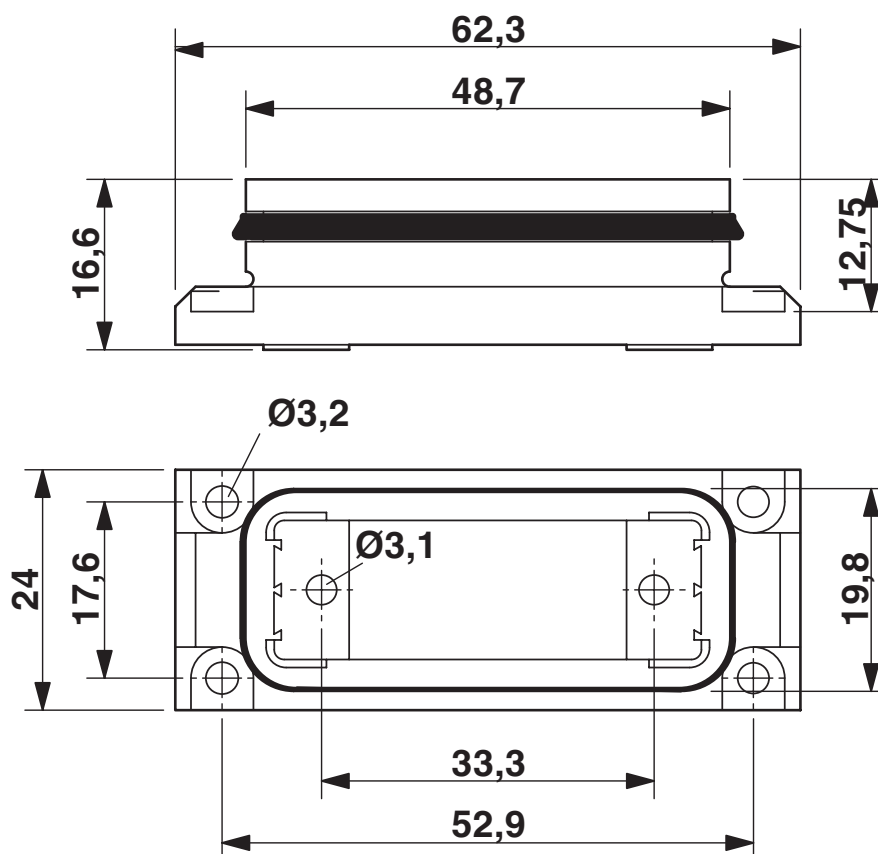
Rysunek wymiarowy
