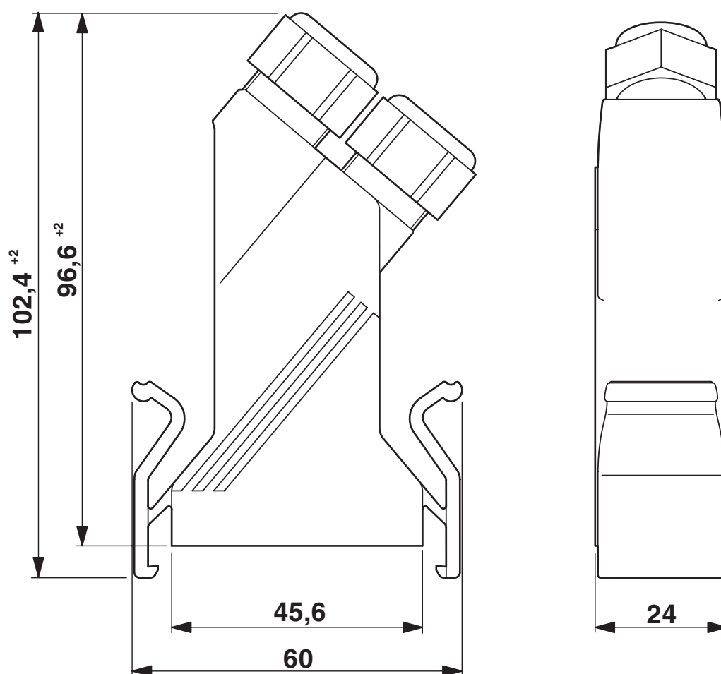
Rysunek wymiarowy
