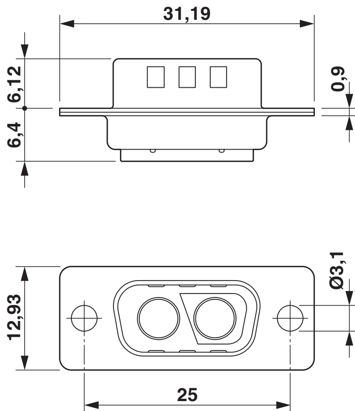
Rysunek wymiarowy
