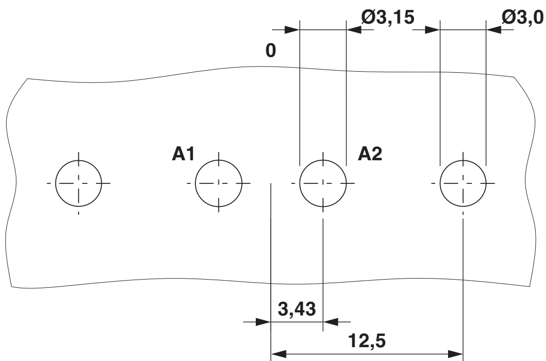
Otworowanie/geometria płytek lutowniczych
