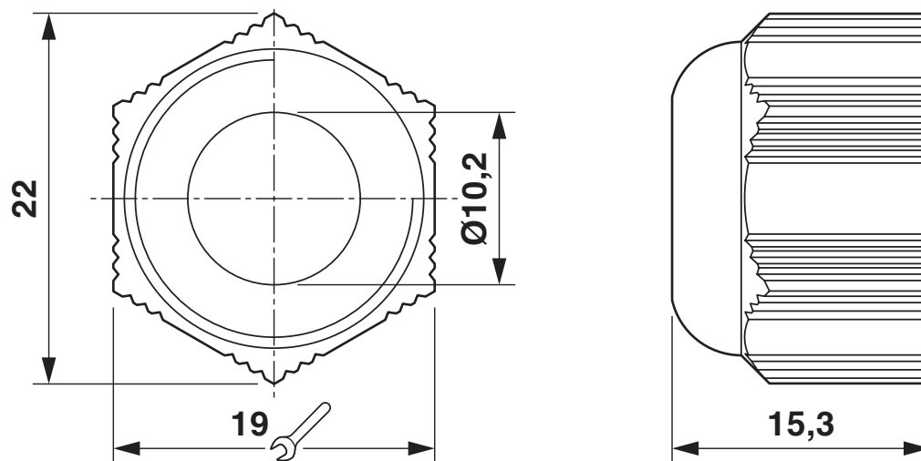
Rysunek wymiarowy
